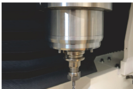
スピンドル
